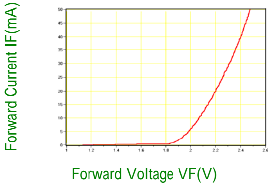
IF-VF(Ta=25 )
